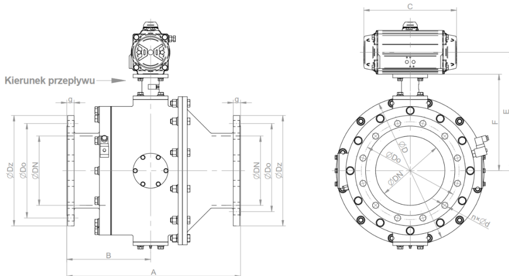
Wymiary zaworu czaszowego „PNEUMOFLEX” w [mm]
